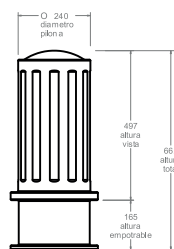
vista alzado
